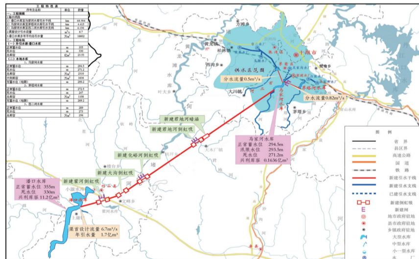
十堰中心城区水资源配置工程平面布置图
