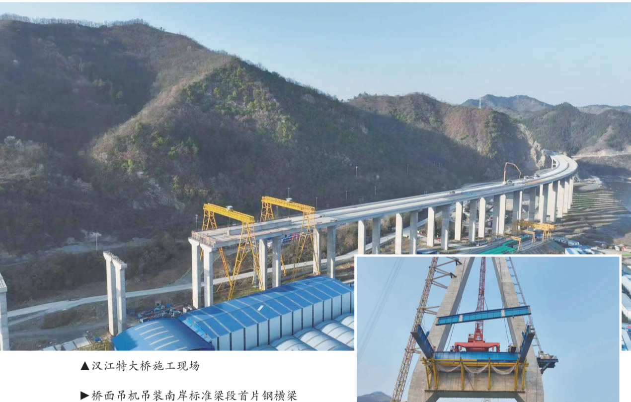
►桥面吊机吊装南岸标准梁段首片钢横梁
